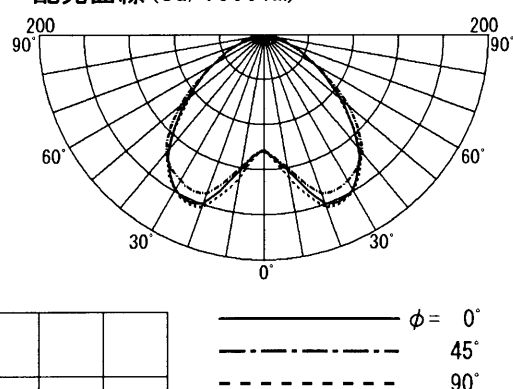
配光曲線 (cd/1000lm)
