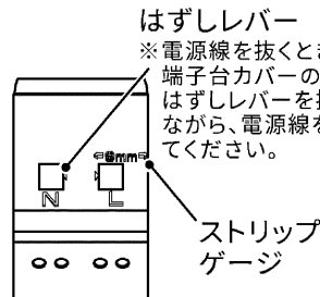
図2 端子台接続
