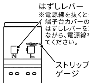
図2 端子台接続
