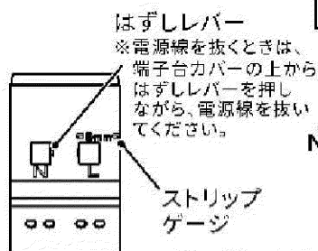
図2 端子台接続
