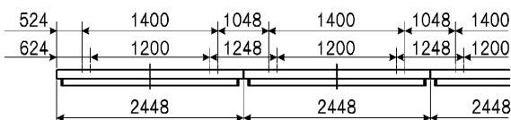
連結寸法図
