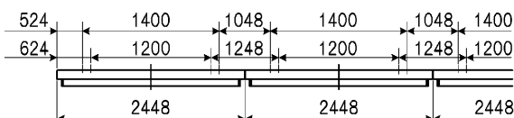
連結寸法図
