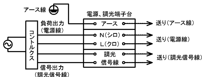
(図10) 調光制御装置との結線図
