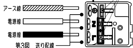
第3図 送り配線
