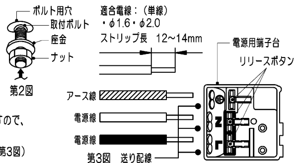
第3図 送り配線
