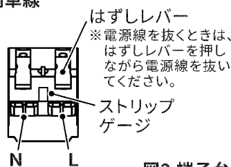
図2 端子台接続
