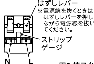
図2 端子台接続
