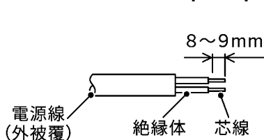
図1 電源線皮むき寸法
