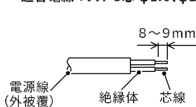
図1 電源線皮むき寸法
