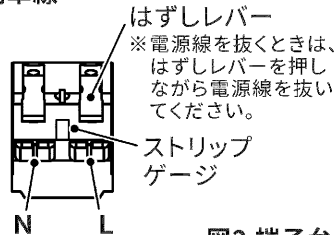
図2 端子台接続
