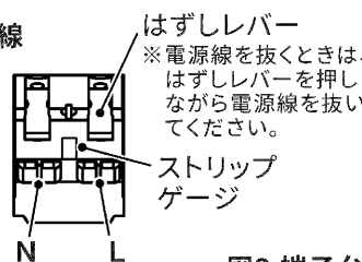
図2 端子台接続
