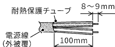
図1 電源線皮むき寸法
