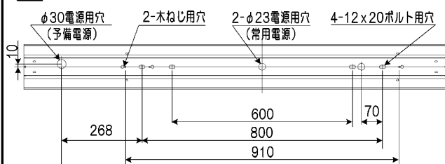
連結寸法図
