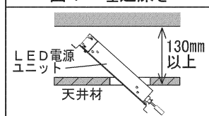
図1 埋込深さ
