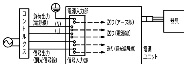
調光制御装置との結線図 (図11)
