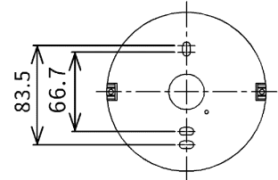
図5 取付寸法図
