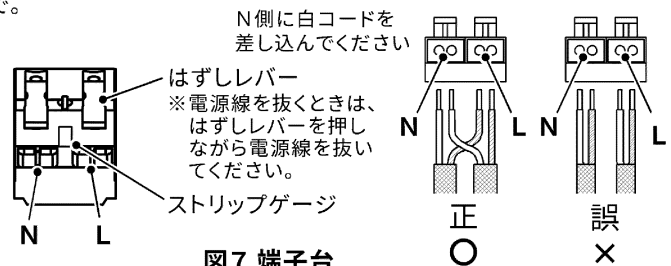
図7 端子台
