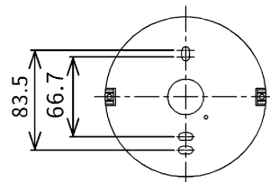
図5 取付寸法図
