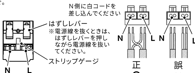
図7 端子台
