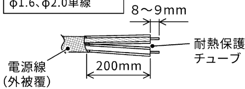
図2 電源線皮むき寸法
