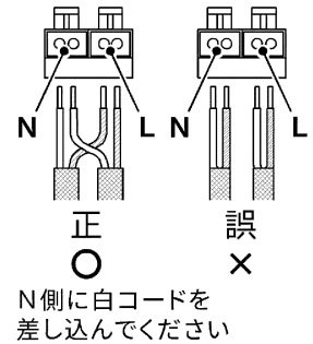
図3 端子台
