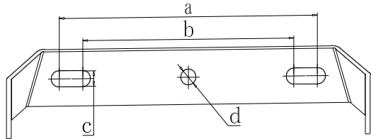
アーム詳細
