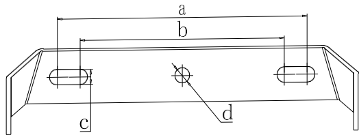
アーム詳細
