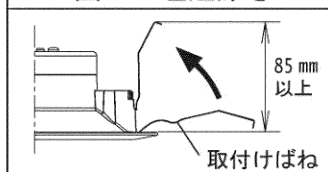
図1 埋込深さ
