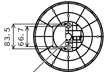
電源線用穴 取り付け寸法図
