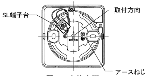
図-4 本体内部
