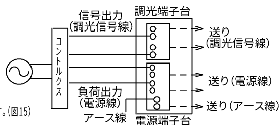
調光制御装置との結線図 (図15)
