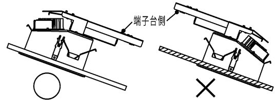
(図8) 傾斜天井に取り付ける場合
