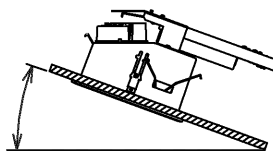
傾斜天井使用時の傾斜角度は10°~30°の間でご使用できます。 ※LEDD-18705M-LD9、LEDD-18706M-LD9のみ取り付けできます。 (図1)
