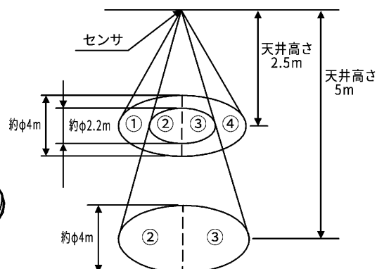
(図15) 床面検知範囲
