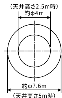
(図15) 床面検知範囲
