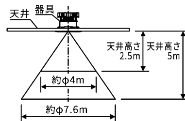
(図14) 天井から床面への検知範囲
