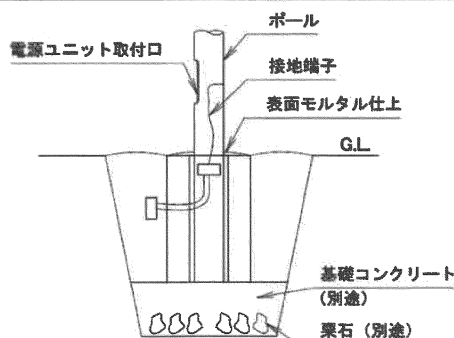
埋込式ポール基礎
