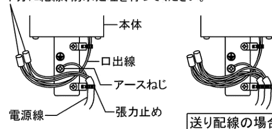
図-3 電源線の張力止め
