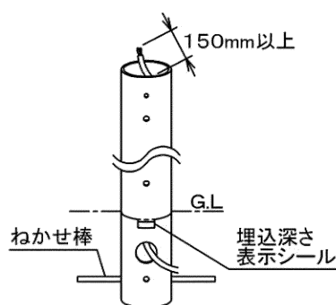
図-2 ポールの埋込み
