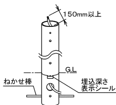
図-2 ポールの埋込み
