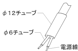
図-3 耐熱保護チューブの取り付けかた
