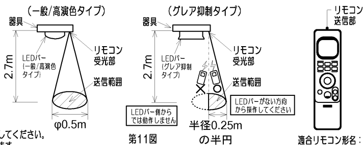
第11図 リモコン送信部 適合リモコン形名: FRC-1825T SET (別売)
