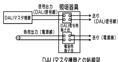
DALIマスタ機器との結線図
