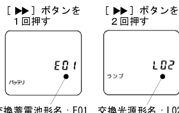
液晶への形名表示(例)
