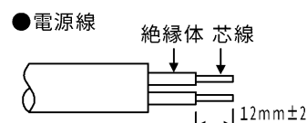
適合電線 φ1.6、φ2.0Cu単線 (図5)
