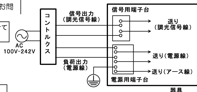
(図8) 調光制御装置との結線図
