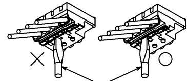
第3図 マイナスドライバー
