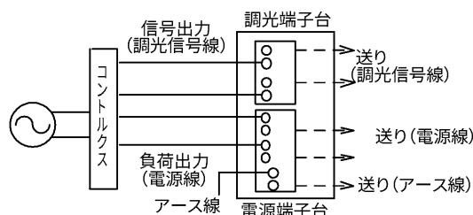
(図19) 調光制御装置との結線図
