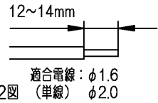
第2図 (単線) 適合電線: φ1.6 φ2.0
