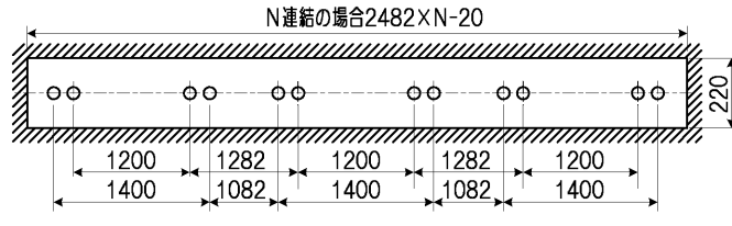
連結取付
