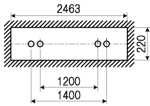
単体取付
