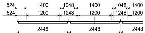
連結寸法図
