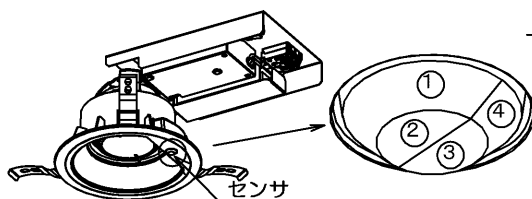
(図12) エリアカットシール貼り付け位置
