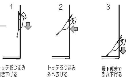
取付け金具の固定方法
