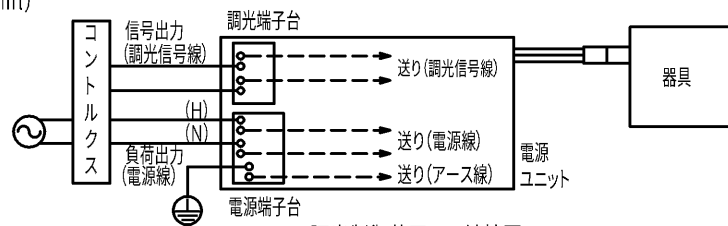
調光制御装置との結線図
