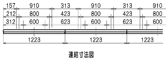
連結寸法図
