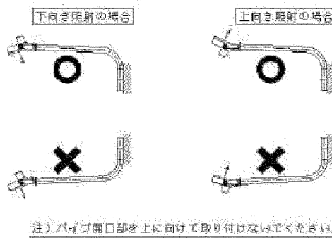
図2 取り付け制限
