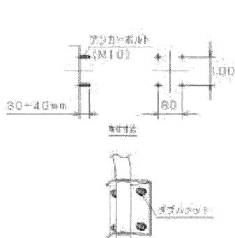
図1 取り付け寸法
