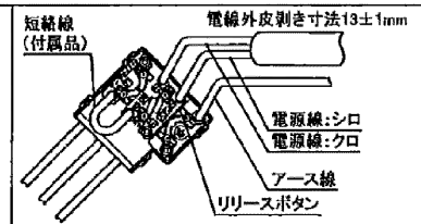
3線引配線の場合(平常時の点滅操作)
