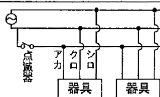
3線引配線の場合(平常時の点滅操作)
