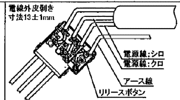
3線引配線の場合(平常時の点滅操作)
