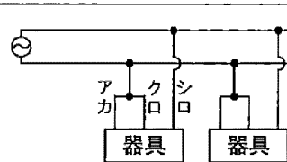
2線引配線の場合(連続点灯)
