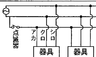
3線引配線の場合(平常時の点滅操作)
