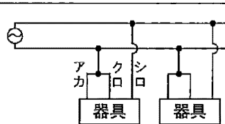
2線引配線の場合(連続点灯)
